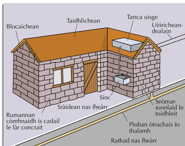
Diagram 8.31b: Taigh ann an sgeama làraichean-is-seirbheisean
