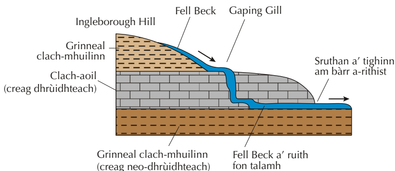
Diagram 4.5: Drèanadh eadar-ùineach
