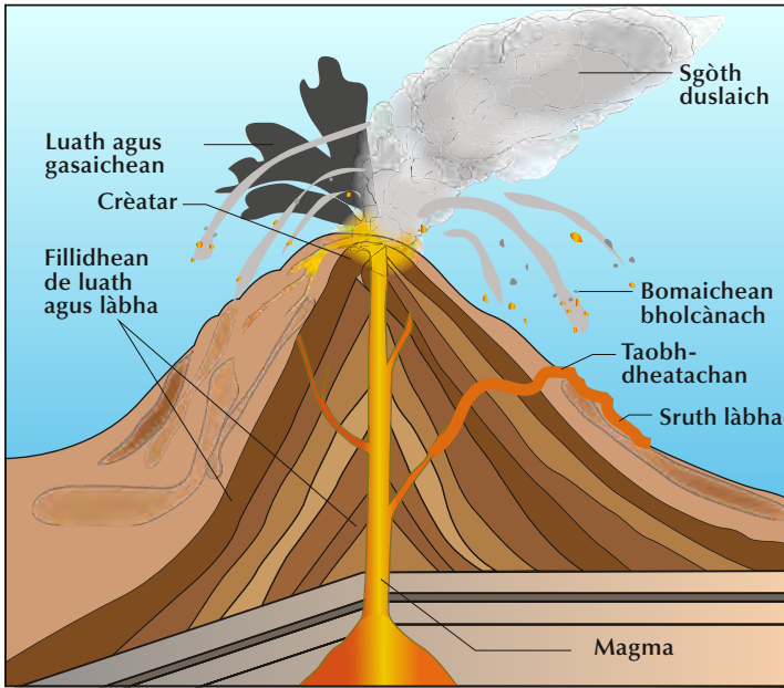
Diagram 11.14: Structur bholcàno
