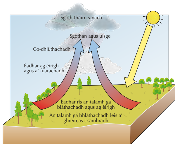
Diagram 10.6: Sileadh conbheacsanach
