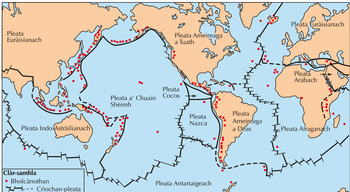
Diagram 11.13: Suidheachadh bholcànothan
