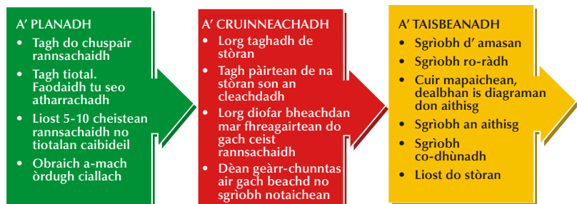
Diagram 1.19: Modail rannsachaidh
