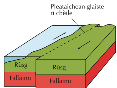
Diagram 11.6: Crìoch-pleata glèidhteach
