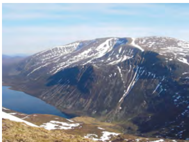
Diagram 5.14: Loch Eanaich
