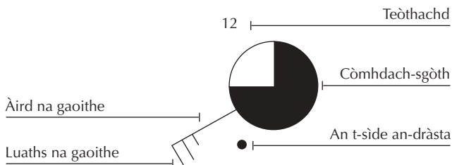
Diagram 2.8: Cearcall stèisean-sìde
