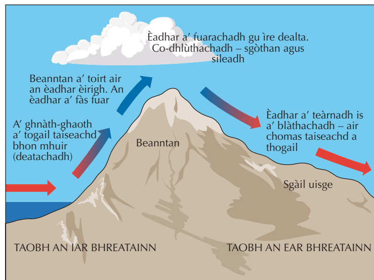
Diagram 2.3: Sìleadh orografaig
